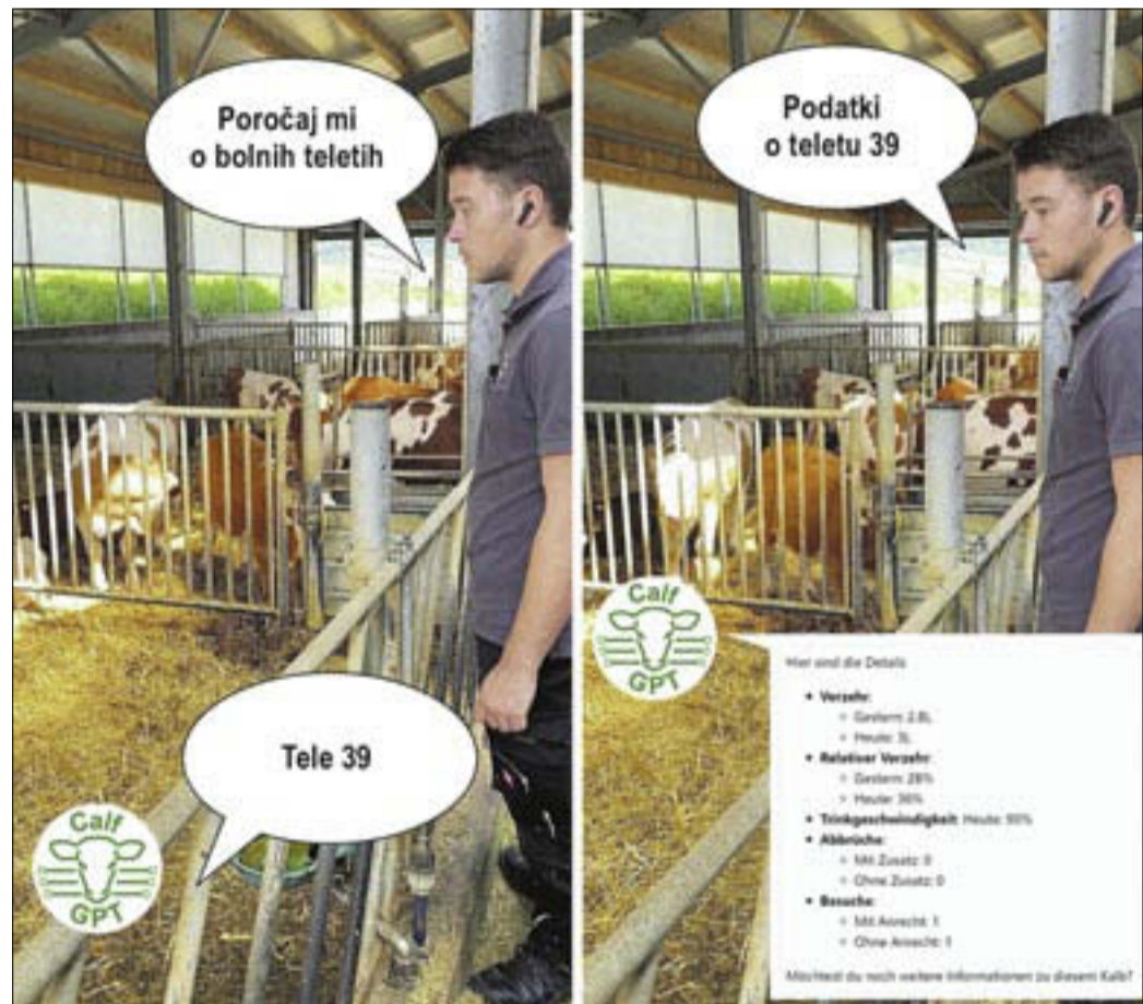
Sistem CalfGPT
